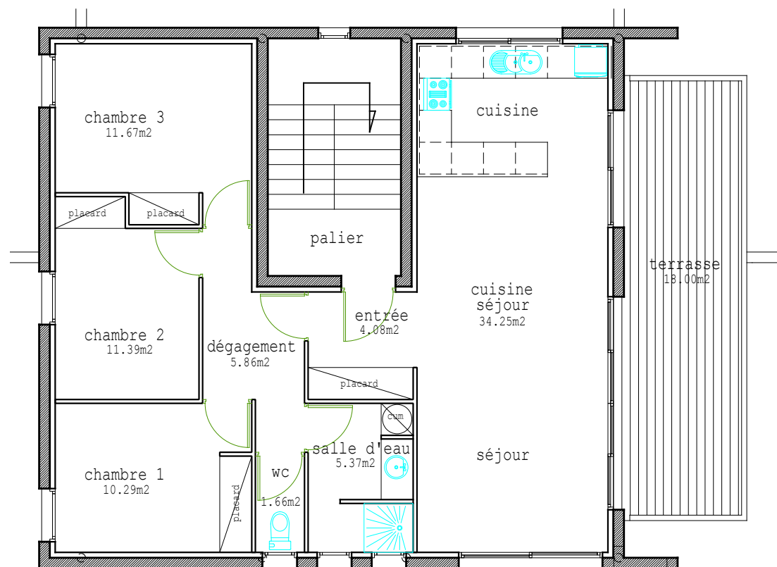
PLAN DE L'ETAGE COURANT appartement T4 SURFACE HABITABLE: 84.57m²
