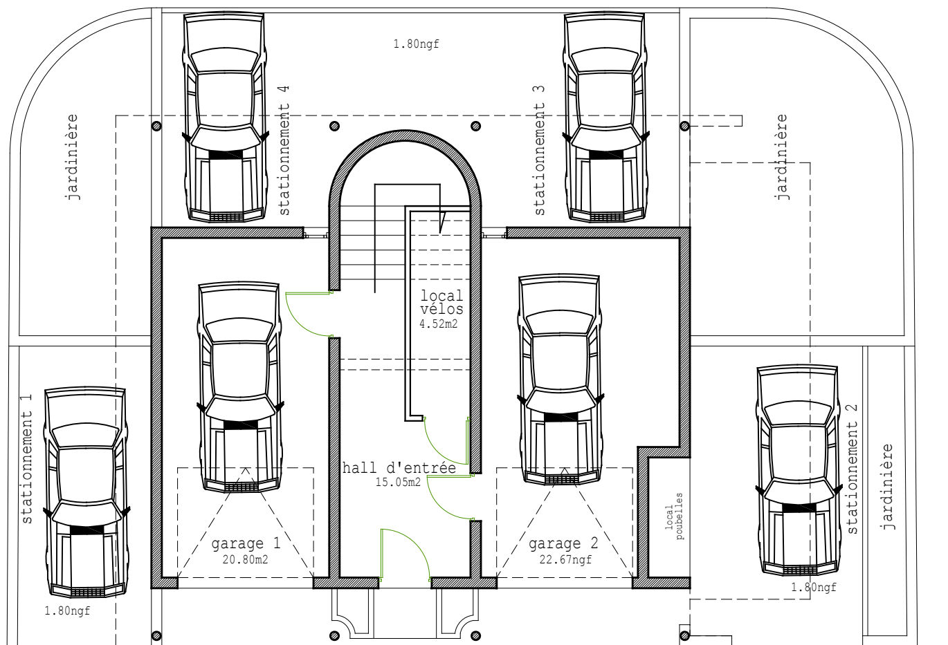
PLAN DU REZ DE CHAUSSEE 2 garages - 1 local vélo
